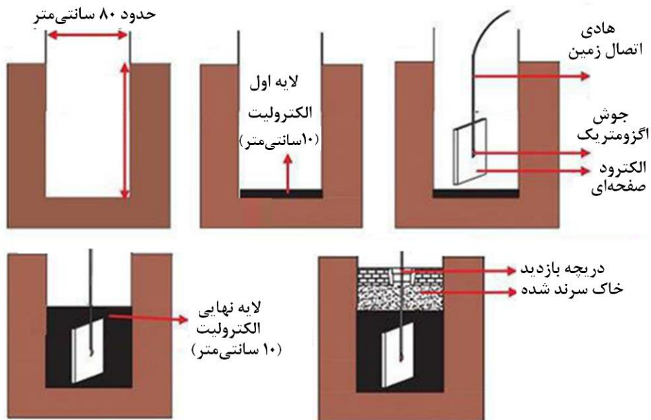
شکل (۲-۹): اجرای الکتروود صفحه‌ای با الکتروولیت
