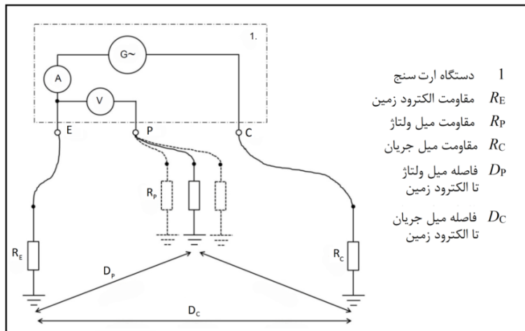
شکل (۱۰): چیدمان الکتروودها به صورت مثلثی
