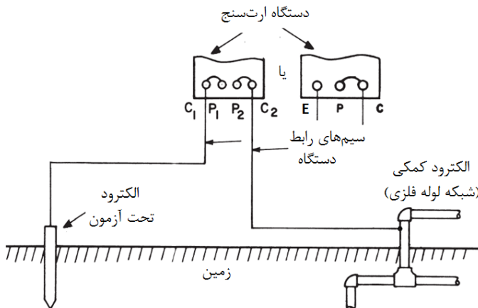
شکل (۱۱): اندازه‌گیری مقاومت الکتروود زمین به روش دوقطه‌ای
